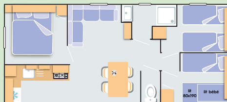
Exemple de plan 3 chambres
